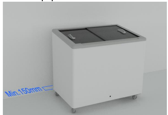
Fig. 5: Distancias mínimas de instalación
